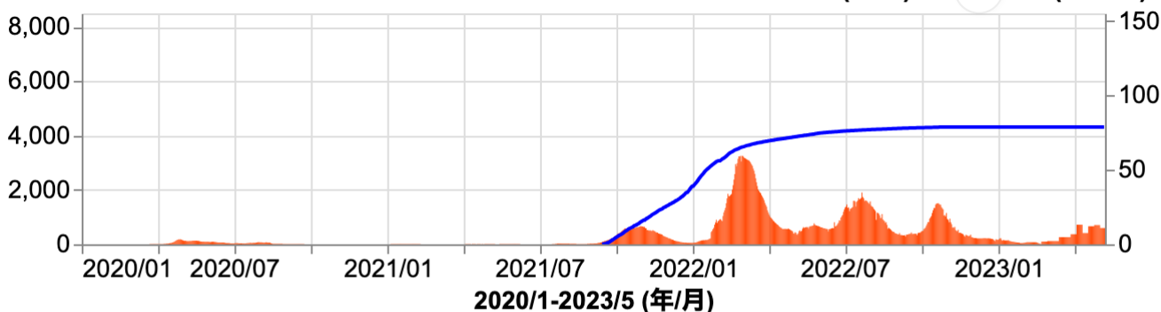
シンガポールの100万人当りの新規陽性者数と100人当りのブースター(追加)接種数累計 (r=0.14)
