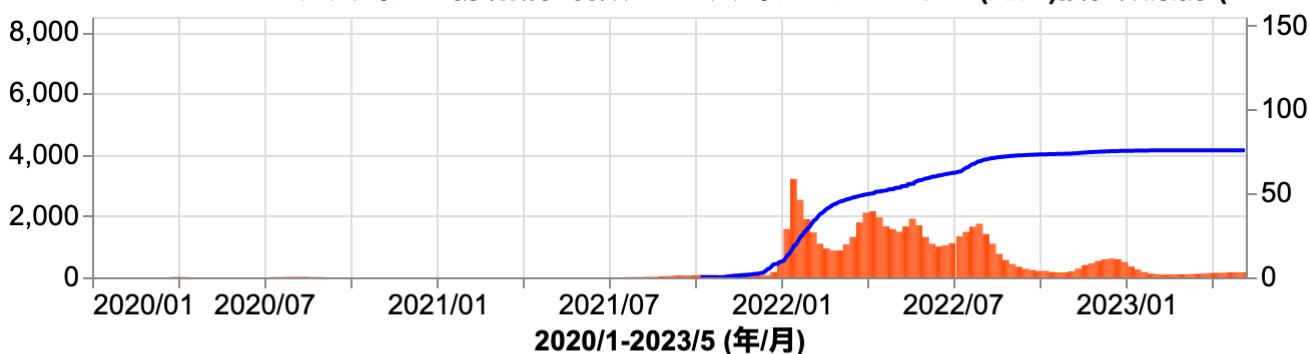
オーストラリアの100万人当りの新規陽性者数と100人当りのブースター(追加)接種数累計 (r=-0.11)
