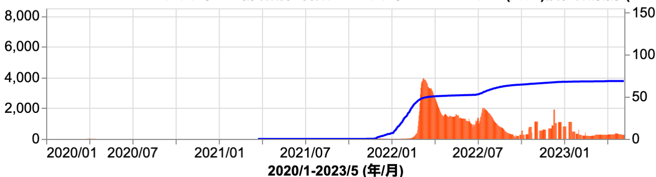
ニュージーランドの100万人当りの新規陽性者数と100人当りのブースター(追加)接種数累計 (r=0.43)
