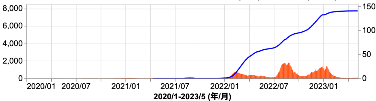
図 4-3-2b: 東アジアとオセアニアがブースター接種開始で感染状況悪化
