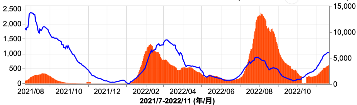
東京都の100万人当りの新規陽性者数と100万人当りの新規接種数 (r=0.45 2022/01/01-2022/11/20)
