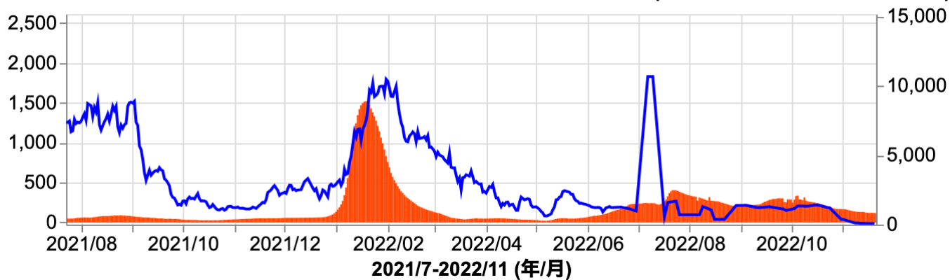
図 4-12-3b: 東京とカタールのワクチン接種と感染状況
